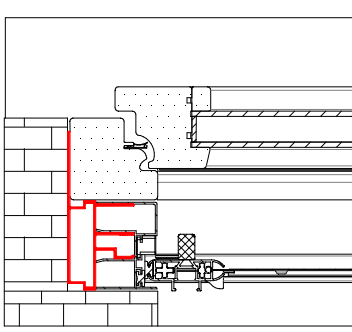
SEZIONE ORIZZONTALE
