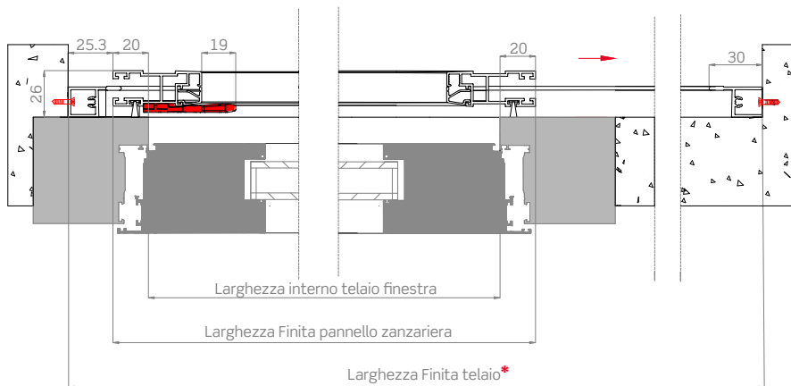
Sezione orizzontale
