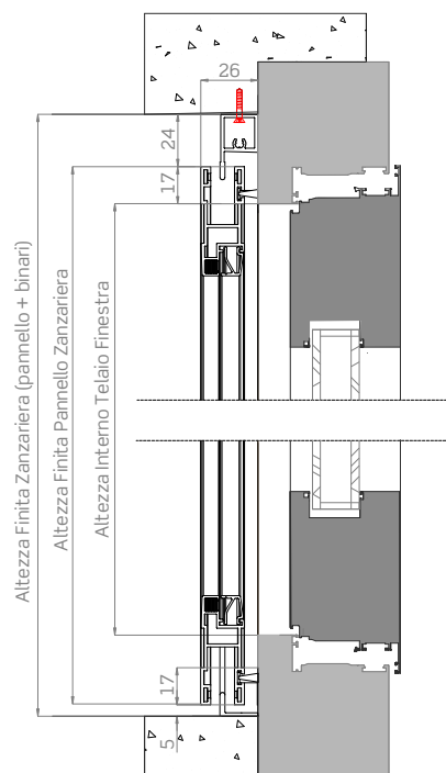
Sezione verticale
