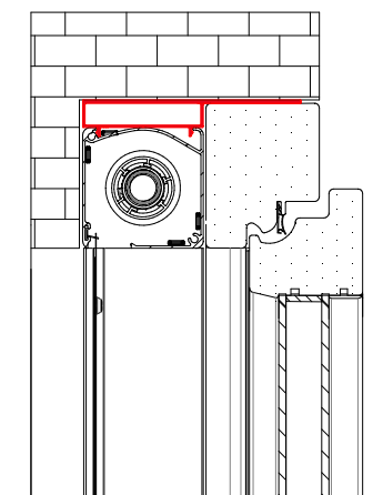
SEZIONE VERTICALE
