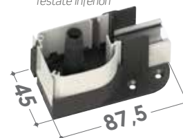
Cassonetto da 42
