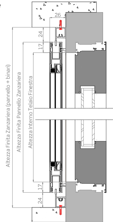
Sezione verticale
