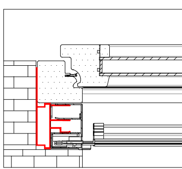
SEZIONE ORIZZONTALE
