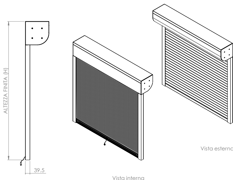
Le immagini rappresentano un esempio di installazione di tipo "A" o "C"
