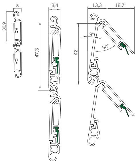
Sezione verticale
