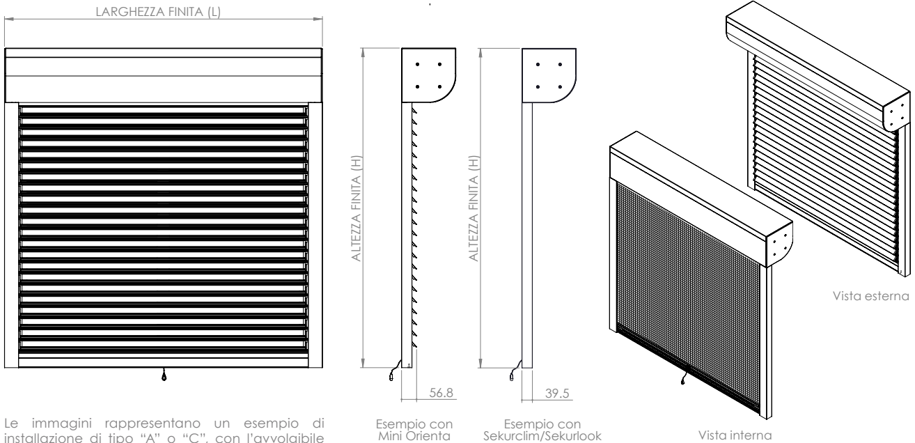
Vista interna
