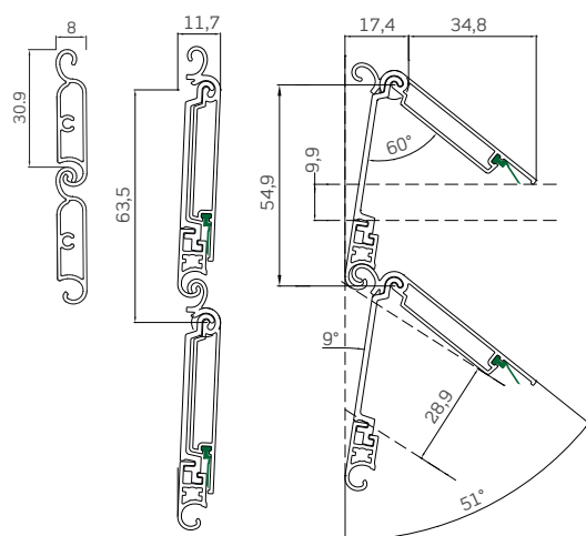
Sezione verticale
