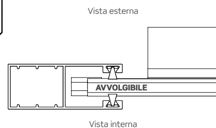
Vista interna
