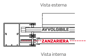
Vista interna
