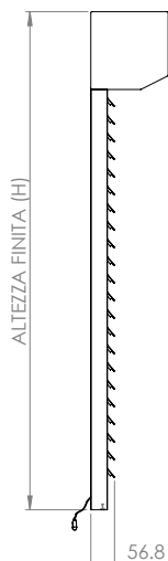
Esempio con Mini Orienta
