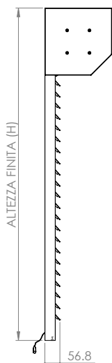
Esempio con Mini Orienta
